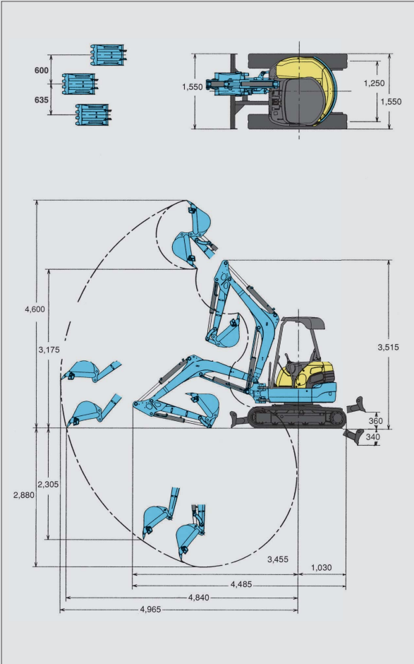
■U30-5 作业范围
